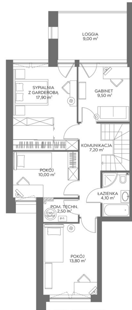
PIĘTRO
